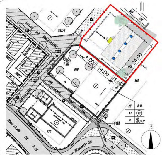
Lageplan
