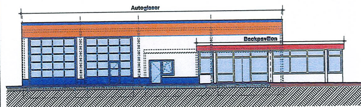
Ostansicht
