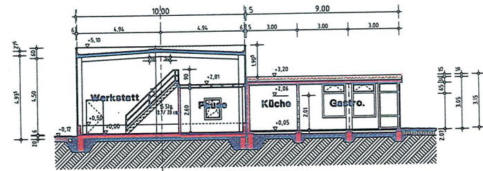
Schnitt A-A
