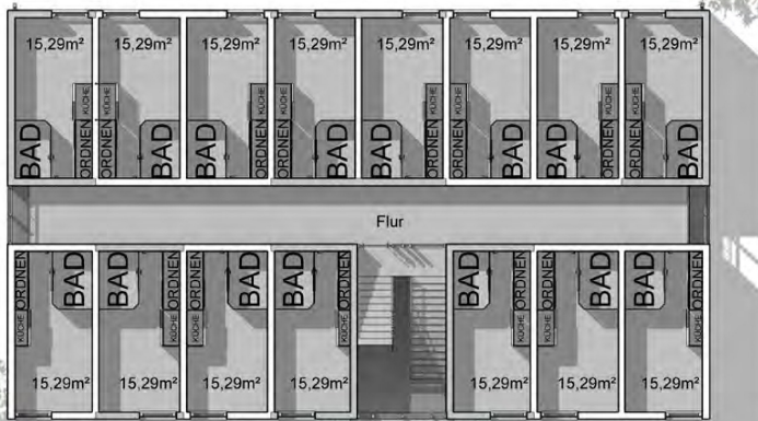
Grundriss
