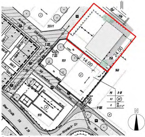
Lageplan
